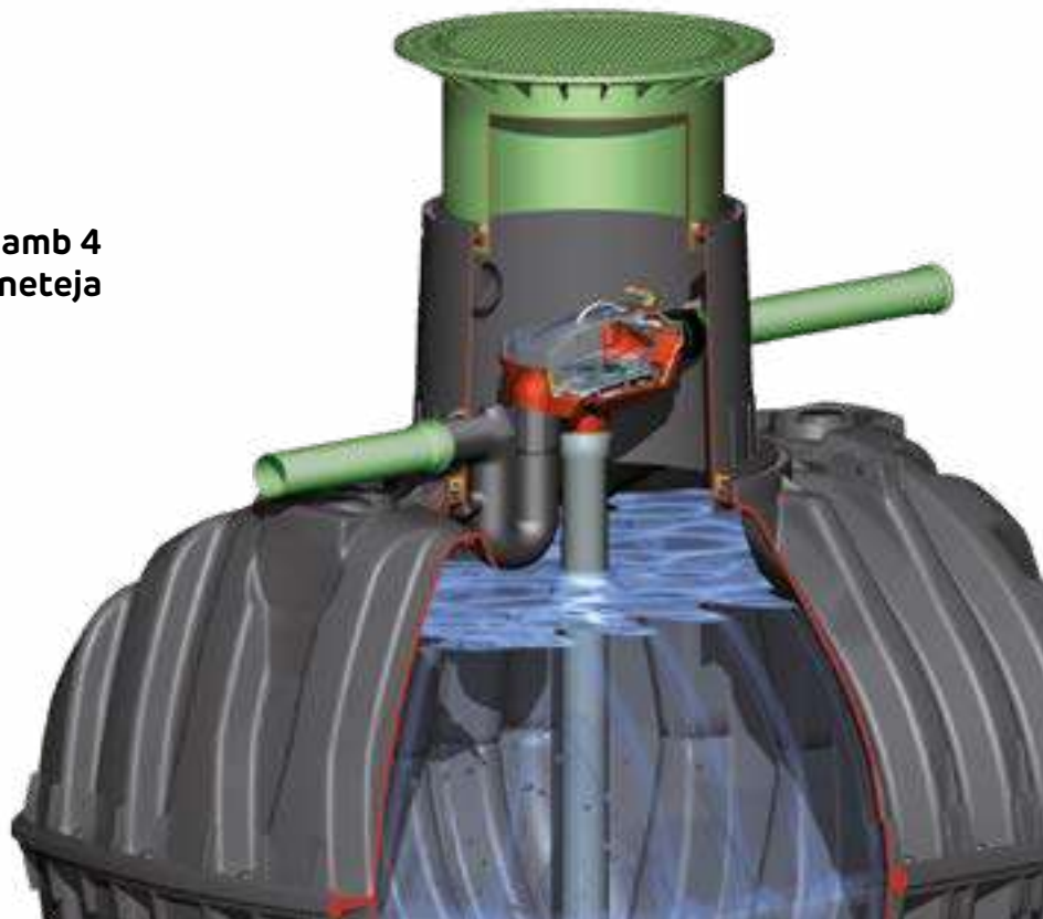
1ª Filtració i first flush
